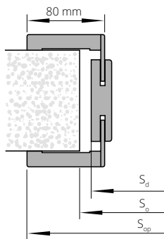
Tunel ZN s obložkami DUO „80“
