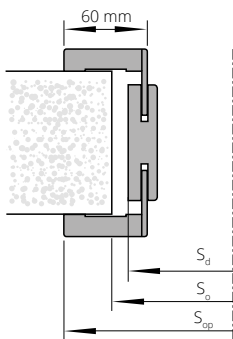
Tunel ZN s obložkami „60“
